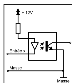
Illustration 3: Schéma interne d'une entrée du lecteur
