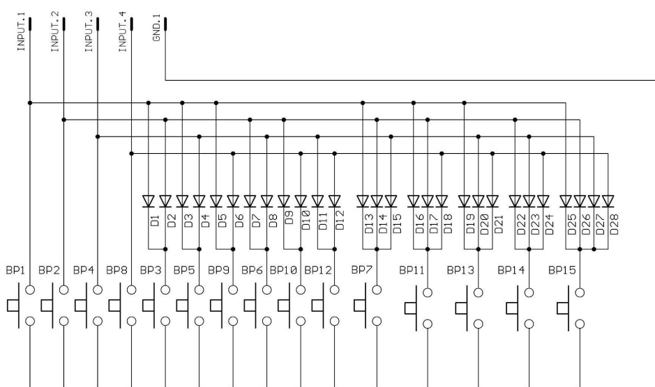
Illustration 3: Schéma interne d'une entrée du lecteur
