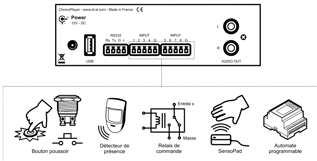
Illustration 1: Exemples de périphériques de déclenchement sur les entrées contact sec
